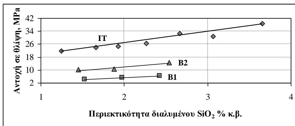
Εικόνα 3. Η αντοχή σε θλίψη των γεωπολυμερών υλικών συναρτίζεται της περιεκτικότητας διαλυμένου \text{SiO}_2 στη σύνθεσή τους.
