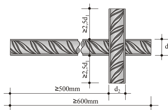
Σχήμα 8-23 Μορφή και διαστάσεις δοκιμίου για δοκιμή διάτμησης
