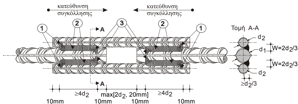
Σχήμα 8-6 Σύνδεση με λωρίδες
