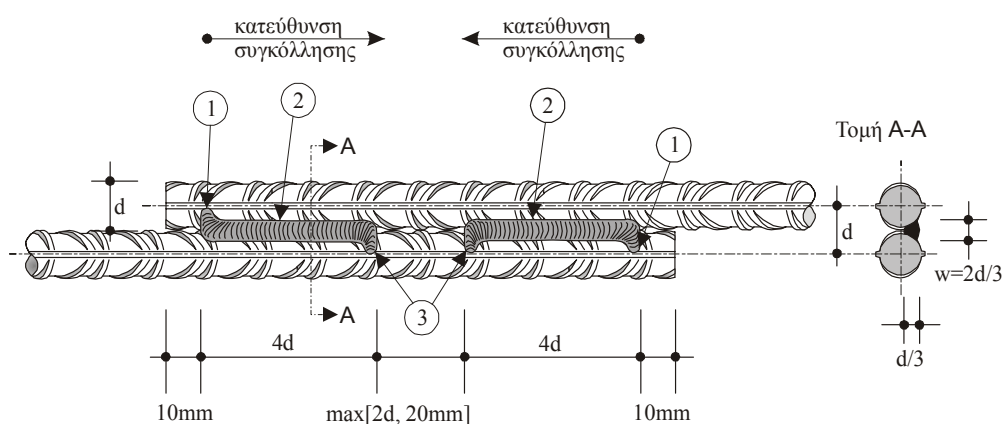
Σχήμα 8-4 Σύνδεση κατά παράθεση με τεχνικές τόξου
