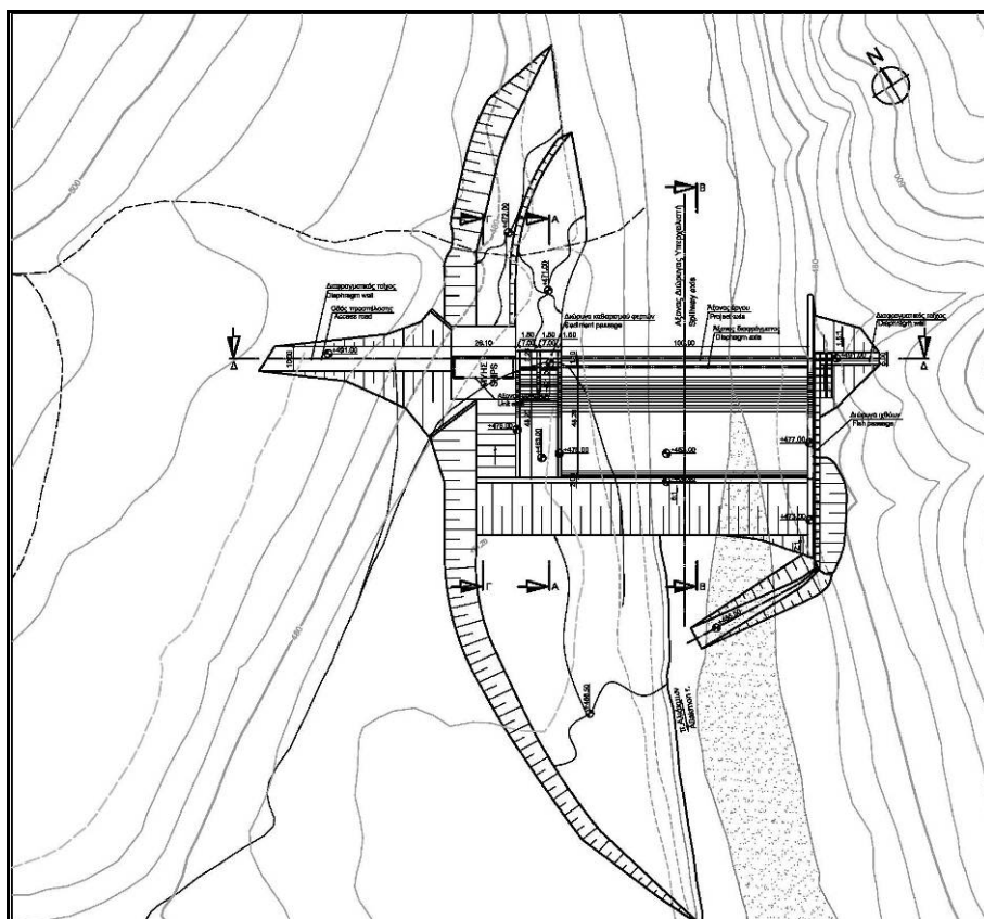
Σχέδιο 6. Γενική διάταξη ΜΥΗΕ Ασπρόκαμπου {3}
