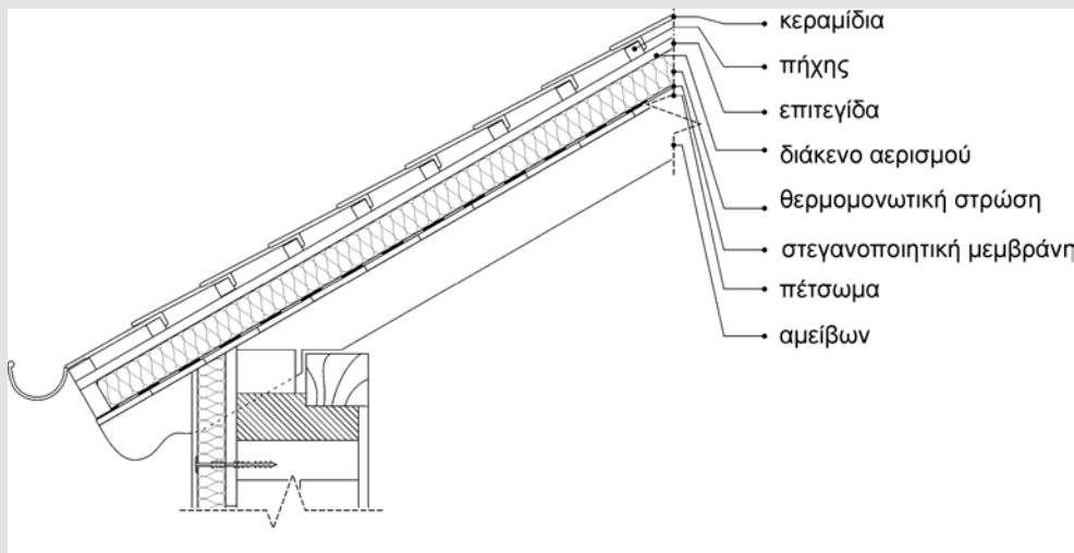
Σχήμα 4.1.5.3β. Διαμόρφωση δικέλυφης (αεριζόμενης) στέγης. Το διάκενο αερισμού διαμορφώνεται μεταξύ της θερμομονωτικής στρώσης και της τελικής επικάλυψης και συμβάλλει στην εκτόνωση των διαχεόμενων υδρατμών.
