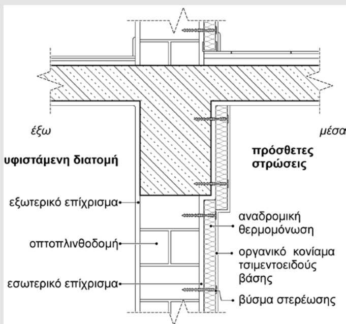
Σχήμα 4.1.3.2. Βελτίωση της θερμομονωτικής προστασίας της τοιχοποιίας με προσθήκη θερμομονωτικής στρώσης από την εσωτερική πλευρά (επικόλληση των θερμομονωτικών υλικών επί της υφιστάμενης τοιχοποιίας και επίχρισή της).
