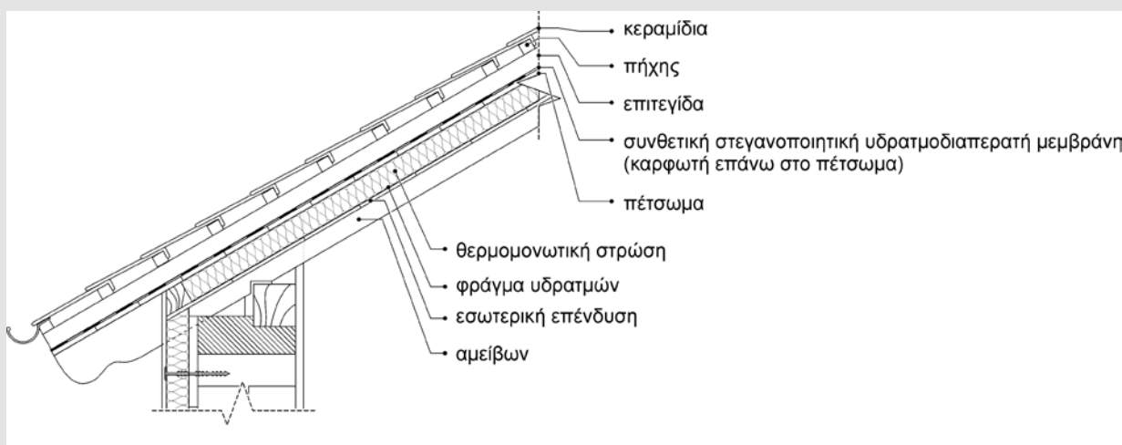
Σχήμα 4.1.5.3α. Διαμόρφωση μονοκέλυφης (μη αεριζόμενης) στέγης με την τοποθέτηση του θερμομονωτικού υλικού ανάμεσα στους αμείβοντες και εσωτερική επένδυση.
