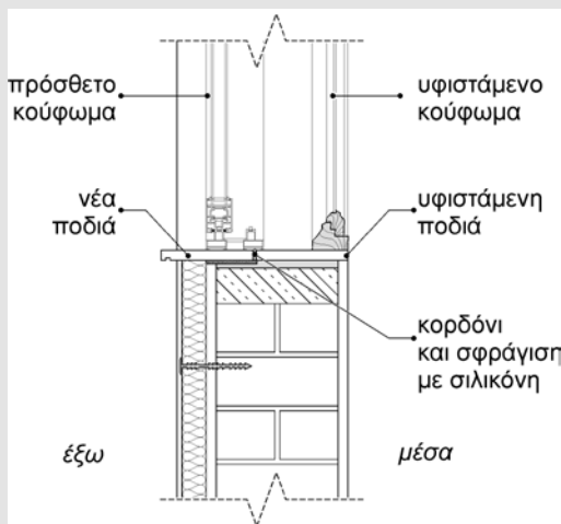
Σχήμα 4.1.9. Βελτίωση της θερμομονωτικής συμπεριφοράς του κουφώματος με τη διατήρηση του υφιστάμενου και προσθήκη και δεύτερου (συρόμενου) εξωτερικά (σχεδόν συνεπίπεδου με την εξωτερική επιφάνεια της τοιχοποιίας).
