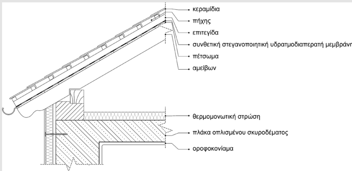
Σχήμα 4.1.5.1. Βελτίωση της θερμομονωτικής συμπεριφοράς μιας οροφής κάτω από μη θερμομονωμένη στέγη με την τοποθέτηση της θερμομονωτικής στρώσης επάνω στην οριζόντια πλάκα.
