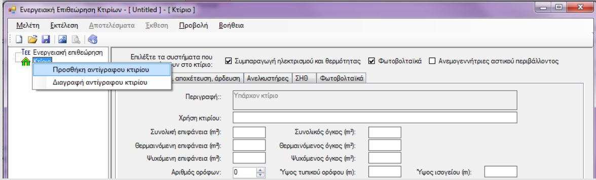
Σχήμα 3.2.3.1. Δημιουργία σεναρίου.
