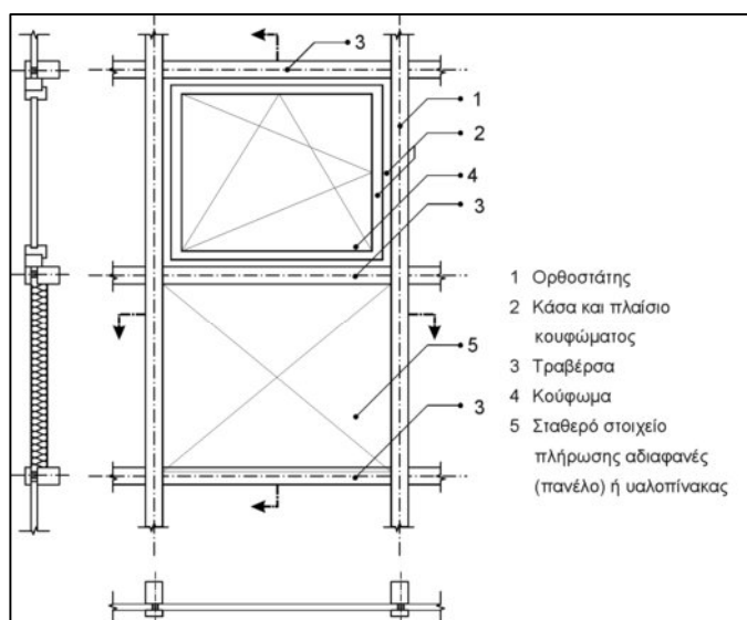
Σχήμα 4. Επιφάνειες τοιχοπετάσματος με διαφορετικές θερμοφυσικές ιδιότητες.
